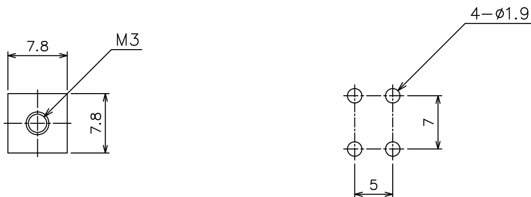
プリント基板用取付穴
